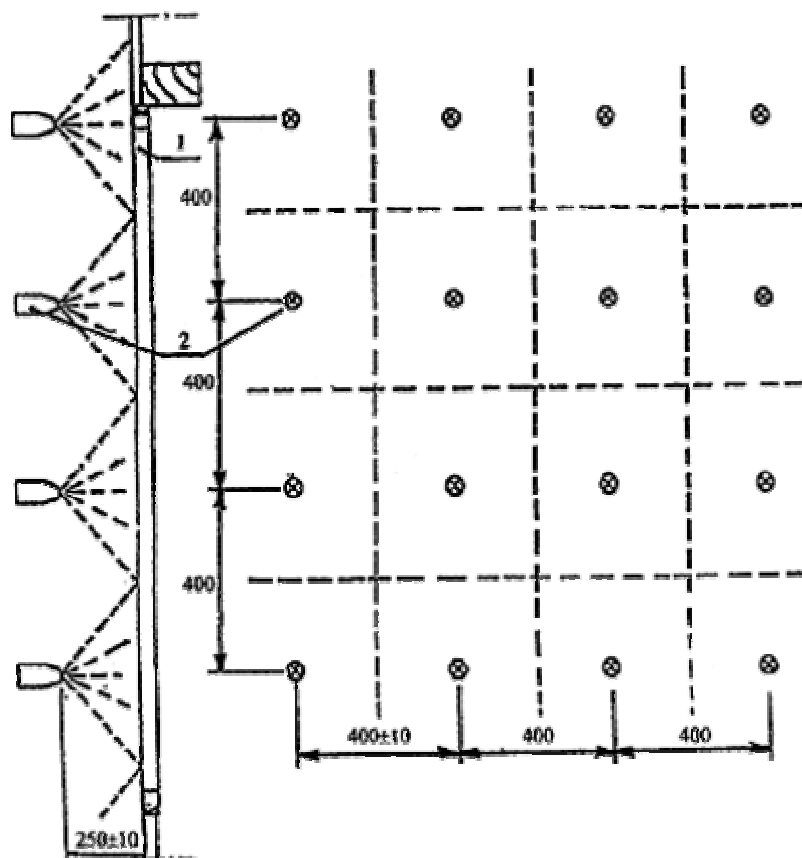
1 - образец; 2 - форсунка дождевальной системы
